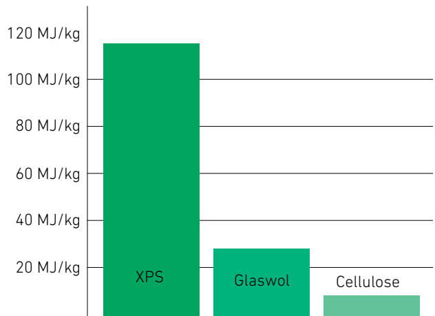
Een vergelijking van het verbruik van primaire energie bij de vervaardiging van isolatiematerialen. Bron: TU Graz
